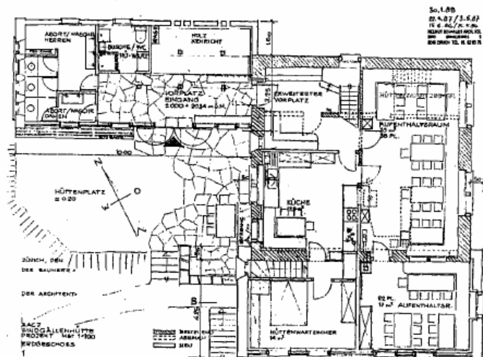
Erdgeschoss Windgällenhütte AACZ H. Schnaudt 30.1.88. (92. JB Seite 21).
