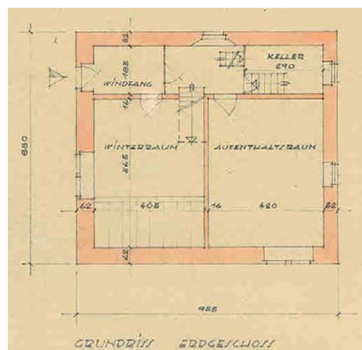
Skizze: Bauaufnahmen der 2. Windgällenhütte 1908 von Hanns-Uli Hohl
